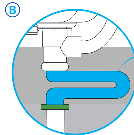
Emboquille bien el desagüe para evitar fugas de agua. Screw the drain well to prevent water leakage.
