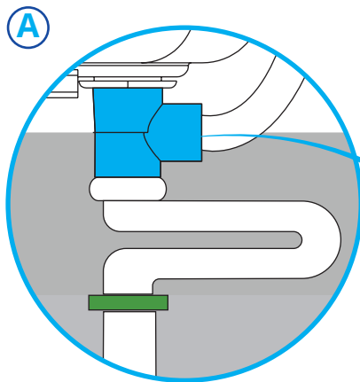
Emboquille bien el desagüe para evitar fugas de agua. Screw the drain well to prevent water leakage.
